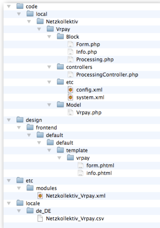
Abb.1.0 Nach dem Entpacken: Inhalt des Ordners „app“
