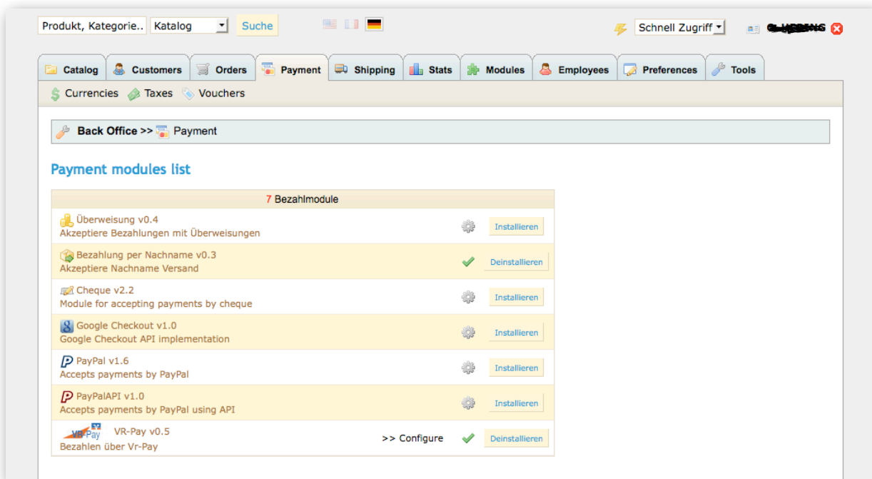
Abb. 2; Zahlungsmodul installieren
